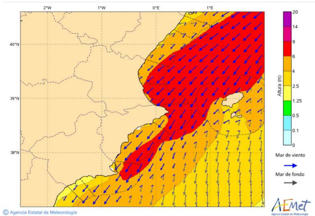
Durísimo temporal marítimo el que se generó la madrugada del lunes 20 al miércoles 22-01-20. Las olas en la zona del golfo de Valencia oscilaron entre los 6 y 8'44m (Fuente: AEMET)
