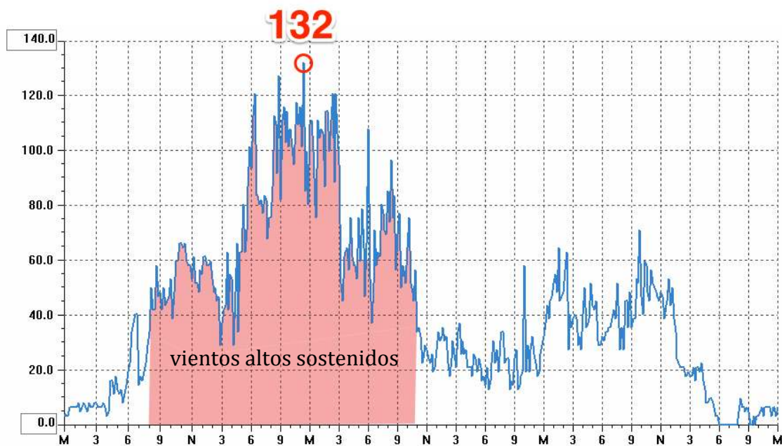
Ráfagas de viento registradas por la estación municipal de ALTEA LA VELLA entre el 19 y el 21/01/20 (en km/h)
